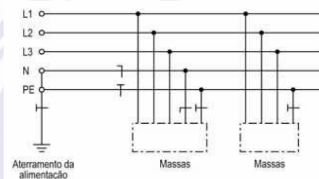
Figura 1 — Esquema TN-S
